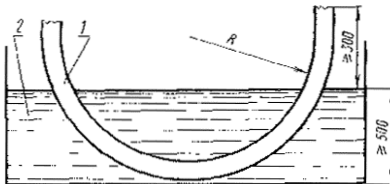
R - радиус изгиба, 1 - образец кабеля; 2 - солевая ванна
