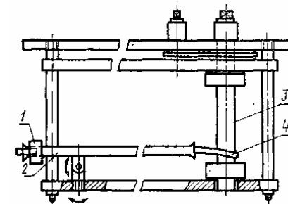
1 — противовес; 2 — труба; 3 — стержень; 4 — образец.
