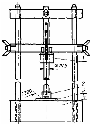
1 — груз; 2 — промежуточная стальная плита; 3 — образец; 4 — стальная плита.
